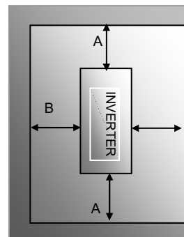
Abstände für die Montage im Schaltschrank
